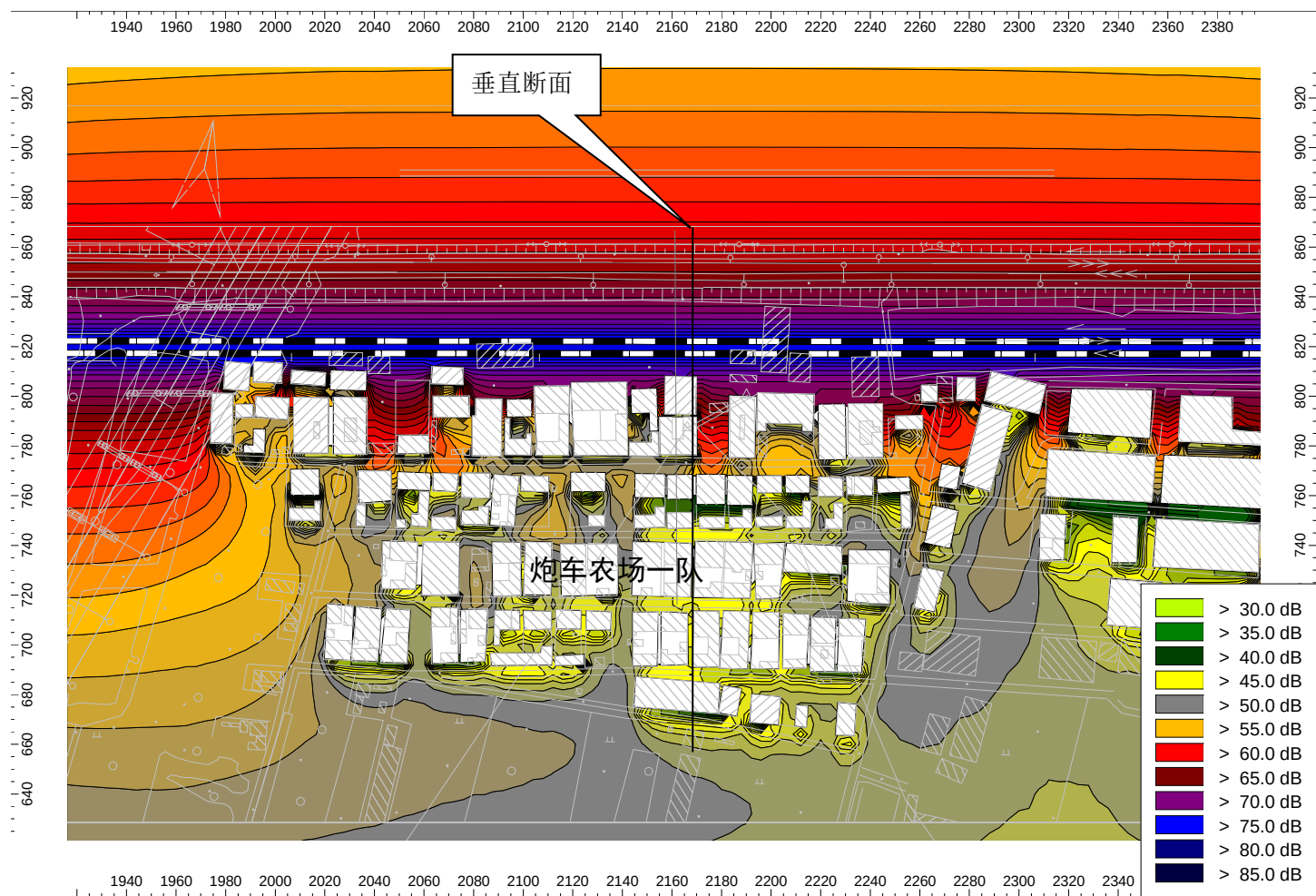
典型路基段（炮车农场一队）近期昼间平面噪声等值线图
