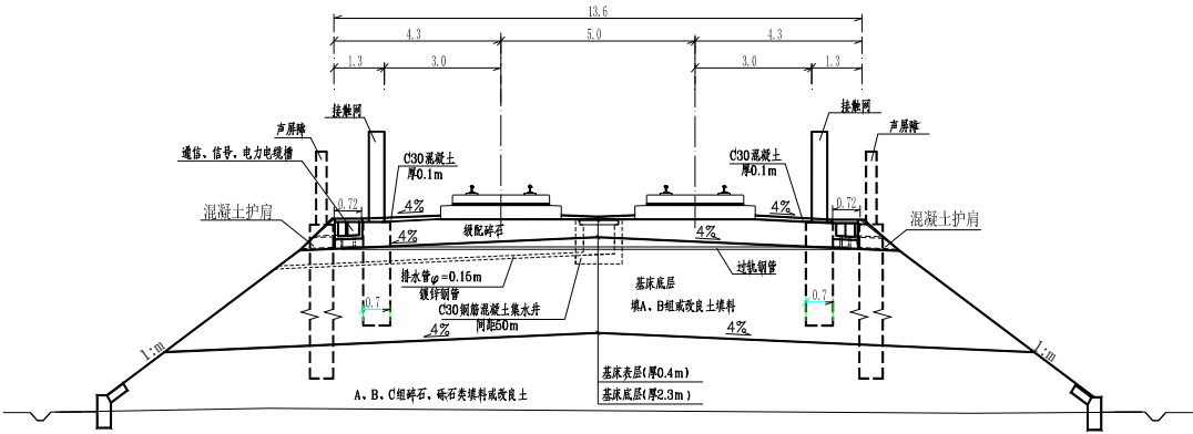
350km/h 双线无砟轨道标准横断面图
