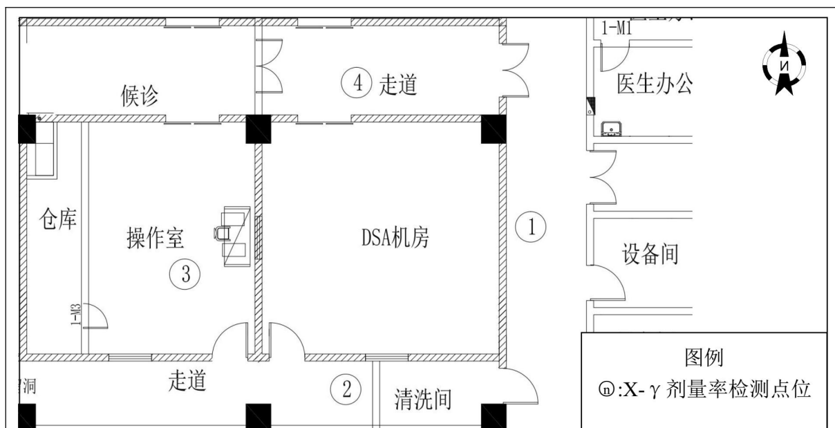
图 8-2 本项目 DSA 机房周围现状检测布点图
