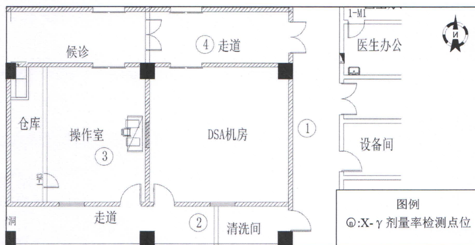
现场检测点位平面示意图
