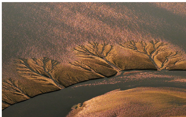
2024年10月29日在盐城市东台条子泥湿地拍摄的潮汐树。
