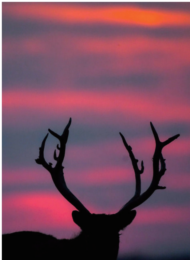
2024年10月28日，在江苏省大丰麋鹿国家级自然保护区拍摄的麋鹿。
